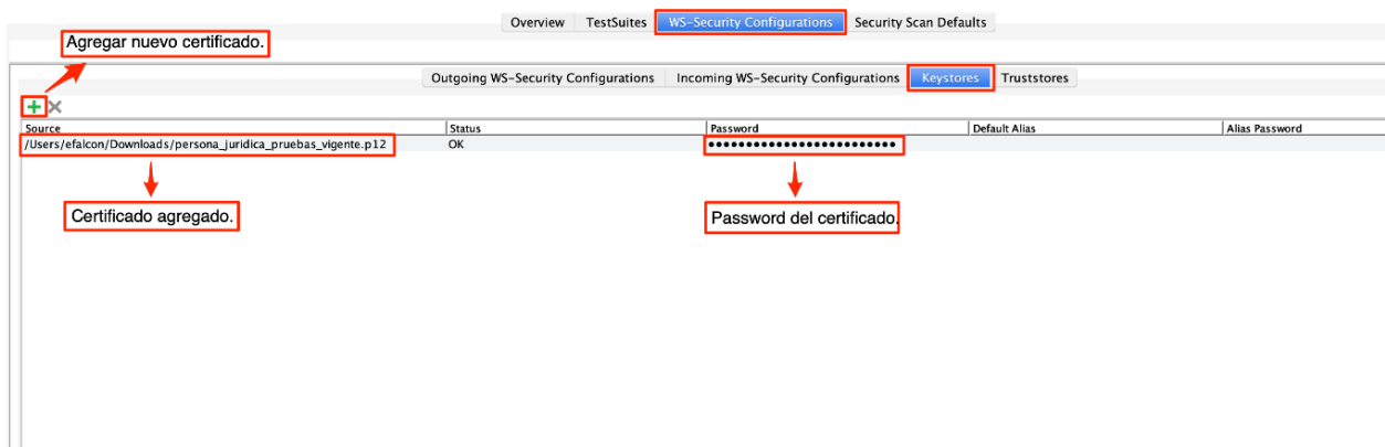
Ilustración 3. Configuración keystore
